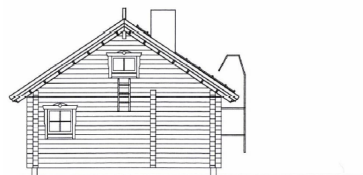
Julkisivu 3
