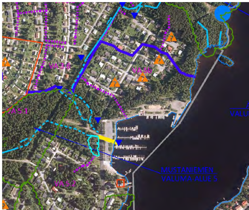
Kuva 13. Kartta hulevesiverkoston nykytilasta. Suunnittelualue sijoittuu Mustaniemen valuma-alueelle (5, kartalla siniset ääriviivat). Suunnittelualueelle sijoittuu laitureiden tuntumaan merkittävä rumpu (keltainen linja) ja hulevesireitin purku (sininen kärkikolmio). Suunnittelualueen pohjoisosassa vihreä alue on "luonnontilainen kosteikko".
